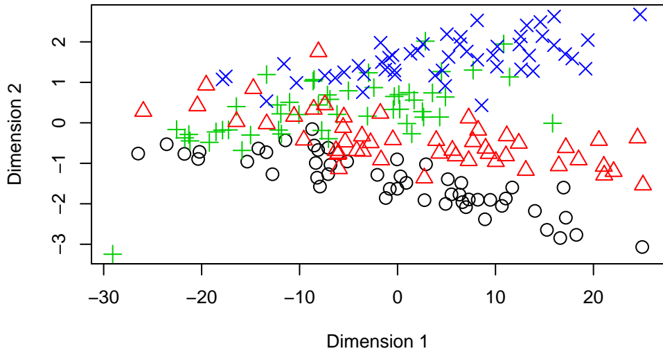
'Sammon Mapping' multidimensionale Skalierung
