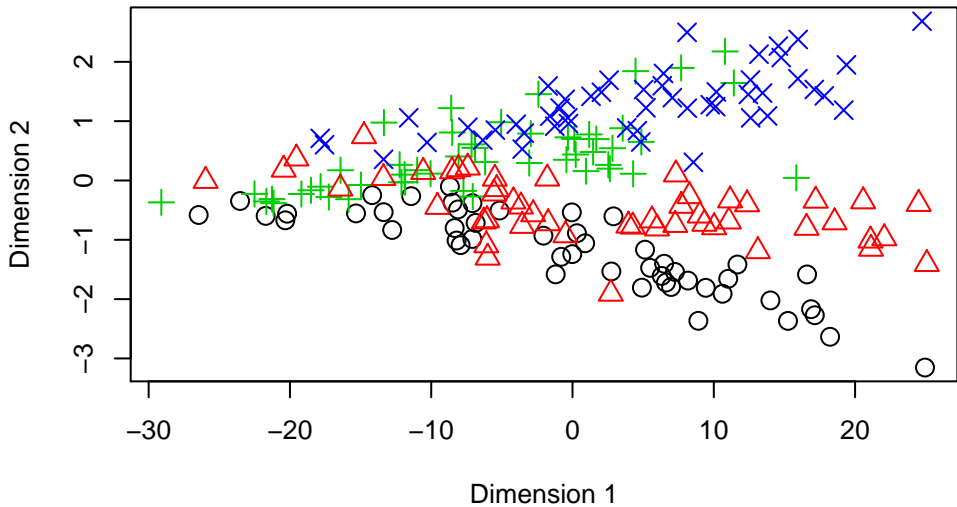
'Isotonic Kruskal-Shepard' multidimensionale Skalierung
