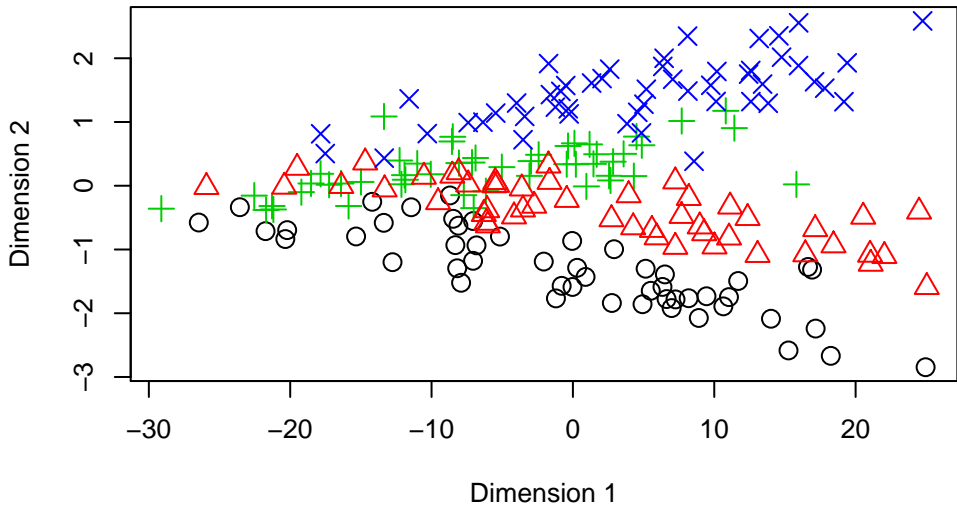
Klassische multidimensionale Skalierung
